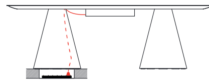
Cable routing inside the base Passaggio cavi all'interno della base
